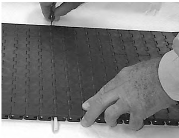
Figura 164: Levante a vareta da esteira
