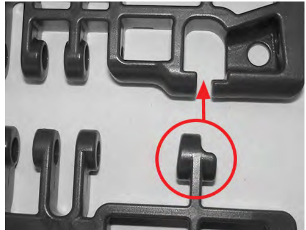
Figura 120: Mova o elo sem vareta no encaixe do elo
